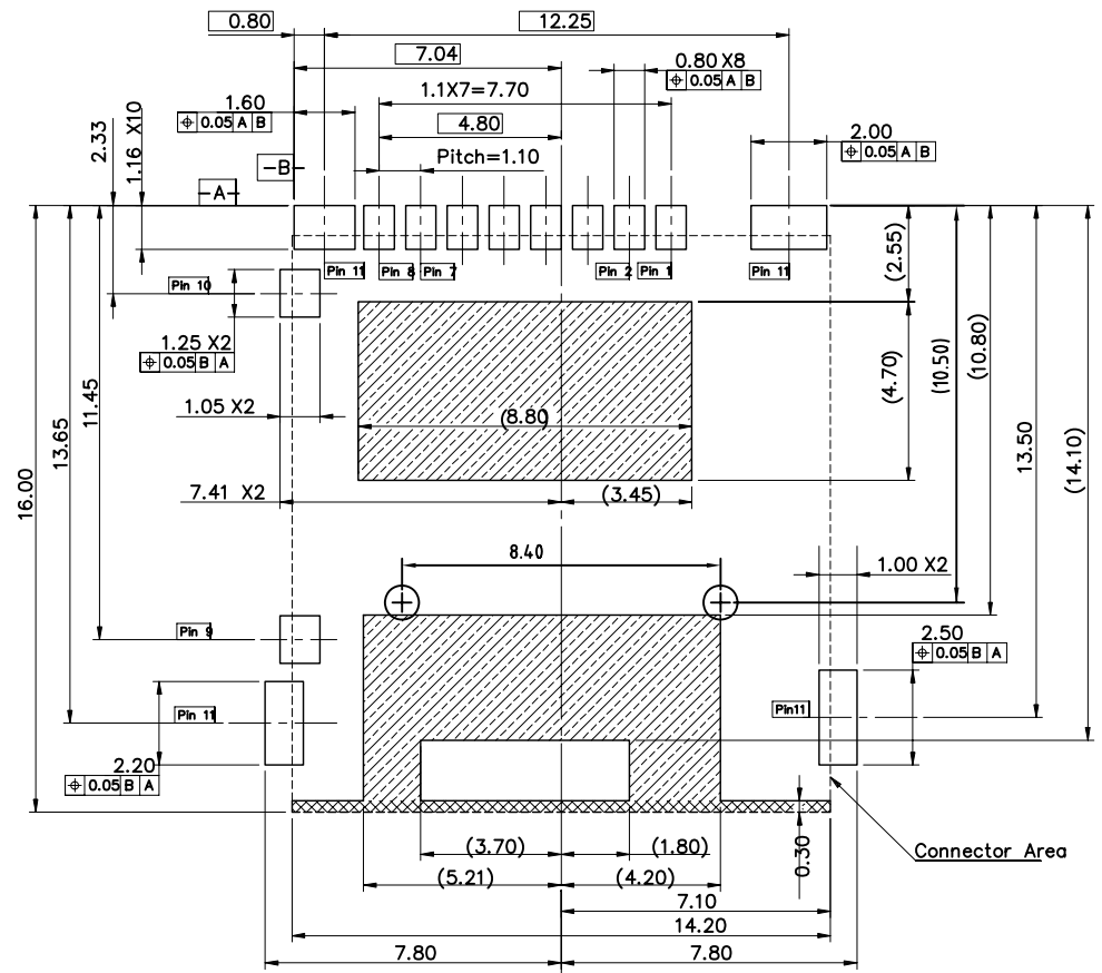
RECOMMEND P.C.B LAYOUT
